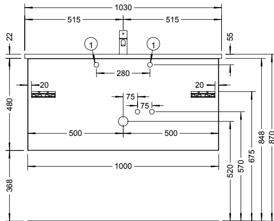
SEZU103/SEZW103/SEZY103
