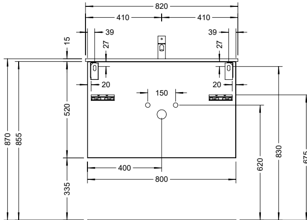
SFGP/SFGR/SFGT082
