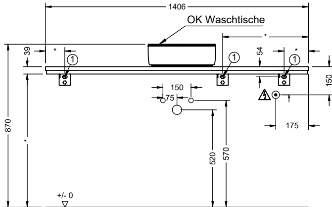
WPGP140 * Maße abhängig von der Planung Finale Maßzeichnung ist mit der Auftragsbestätigung verfügbar!
