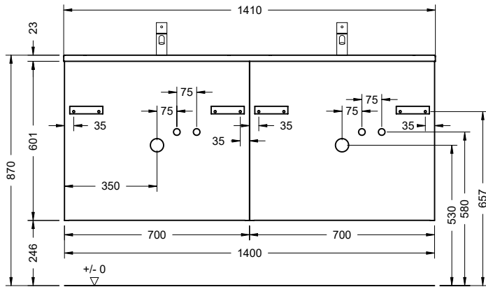
WVAF140
