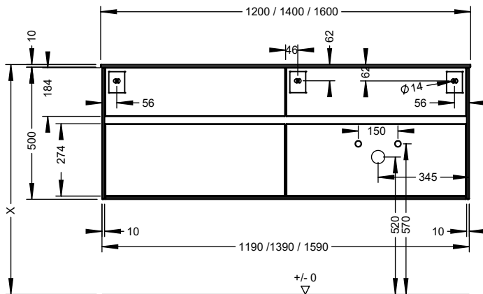
SGGG120R, SGGG140R, SGGG160R X = abhängig vom Waschtisch SGGF120R, SGGF140R, SGGF160R
